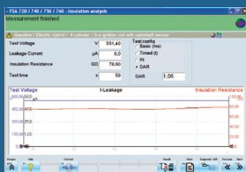
Проверка изоляции
